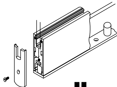
Modulschiene für Seitenteil
