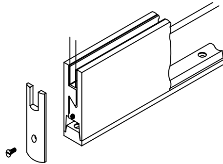
Massivschiene für Seitenteil
